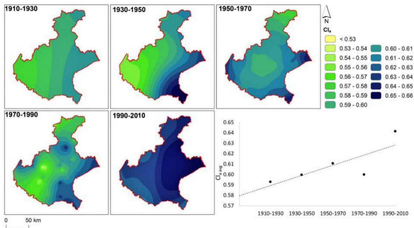
Figura 02.02. Concentrazione delle precipitazioni ( CI_a ) per i diversi tempi e andamento valore medio. [Fonte: Sofia et al., 2017]
