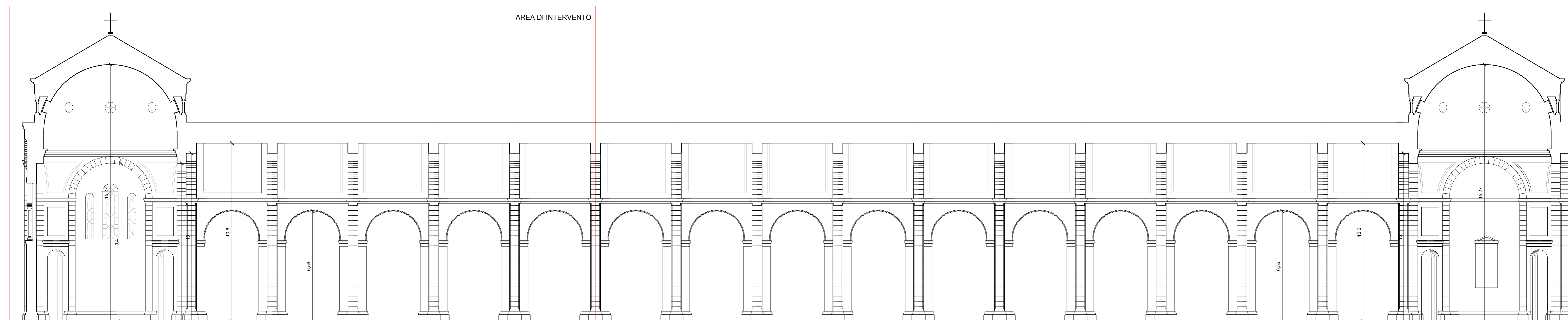
Sezione F - F scala 1:100
