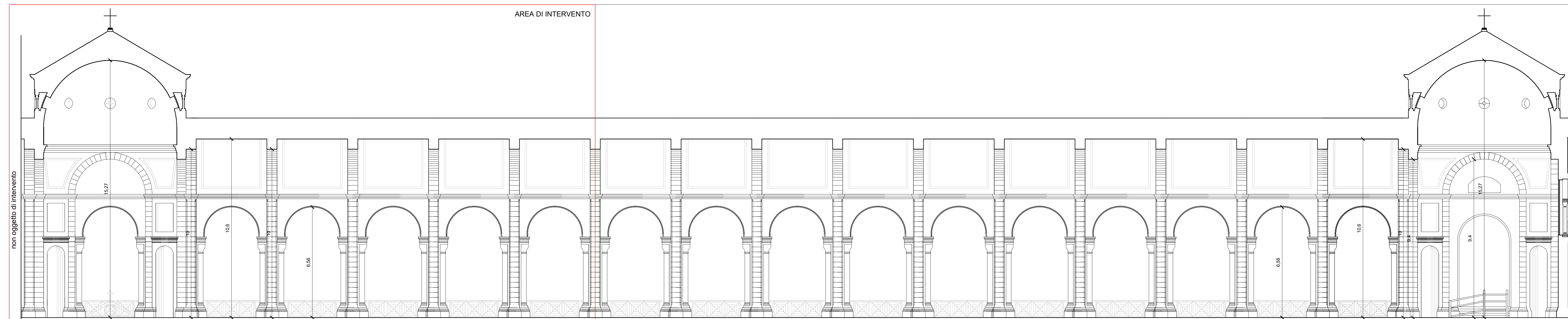
Sezione E - E scala 1:100
