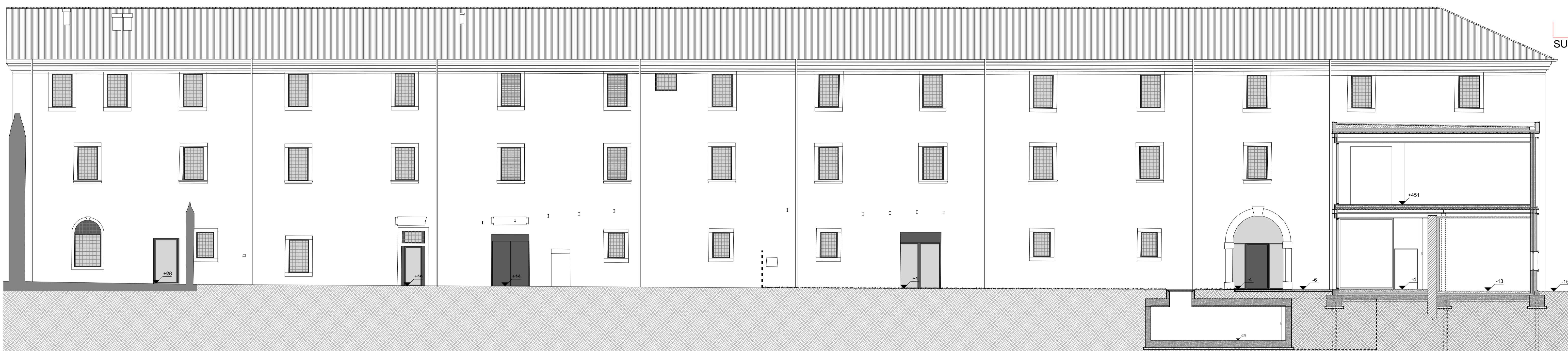
prospetto sud_ SCALA 1:100
