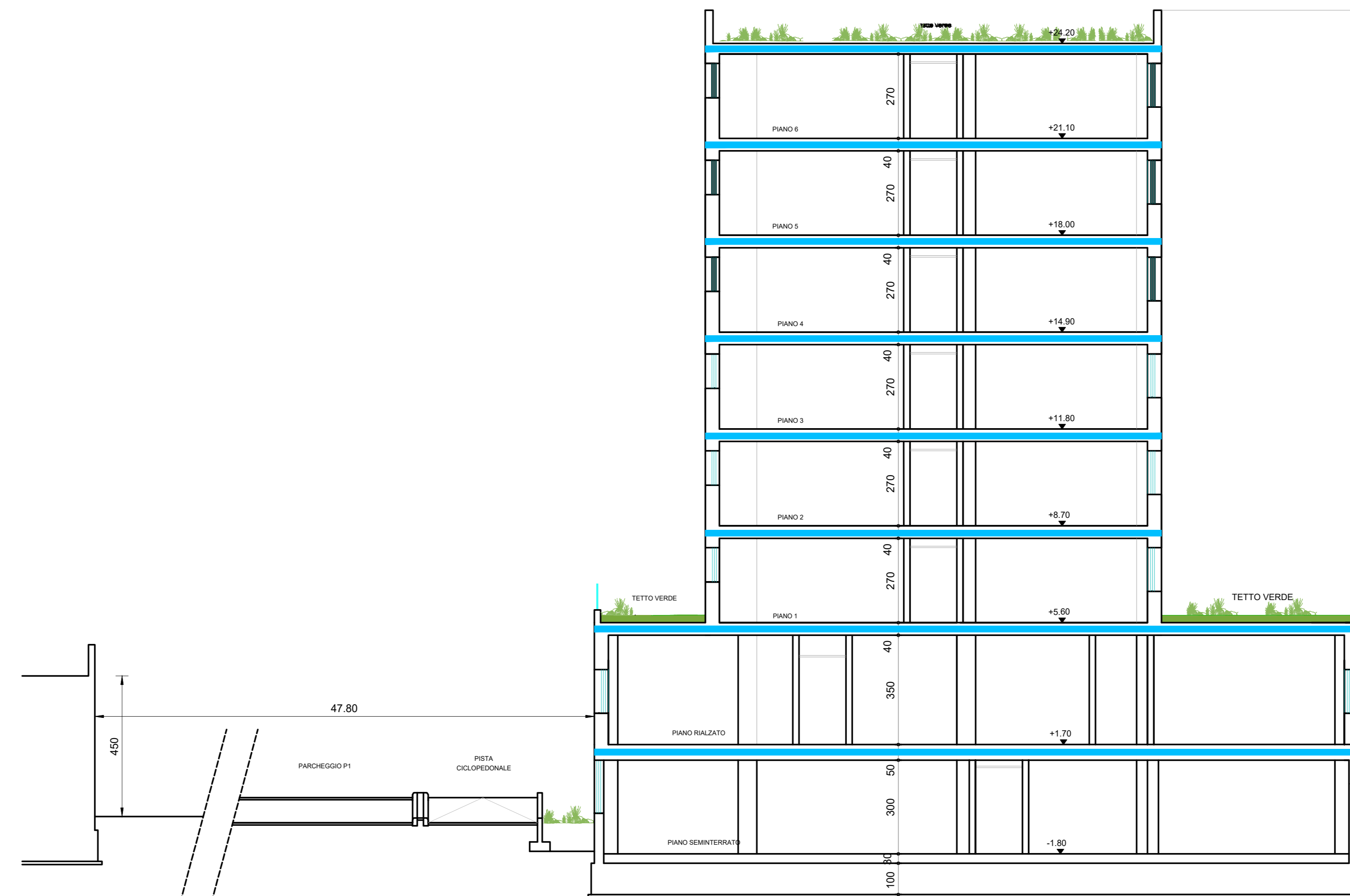
SEZIONE C-C
