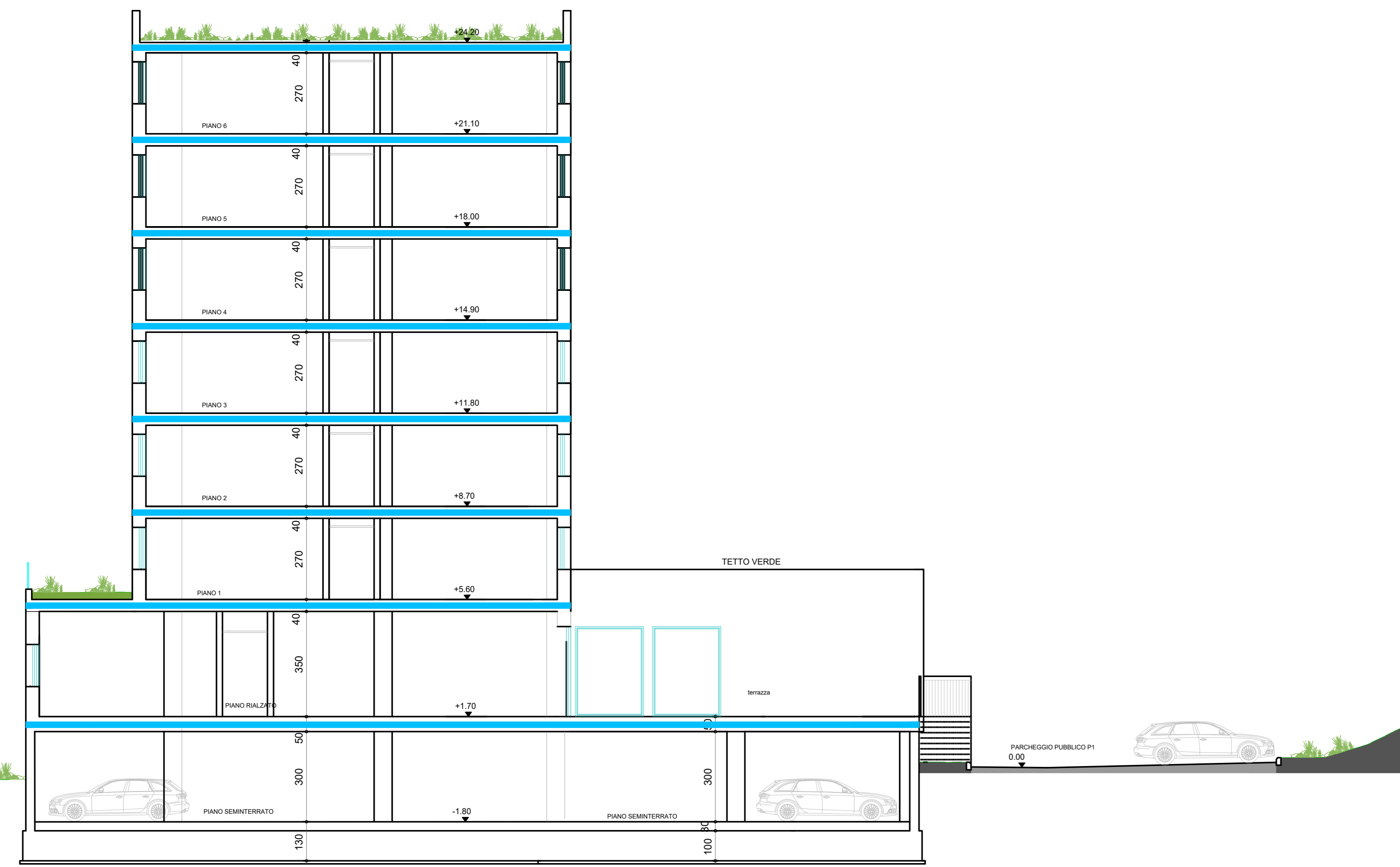
SEZIONE A-A
