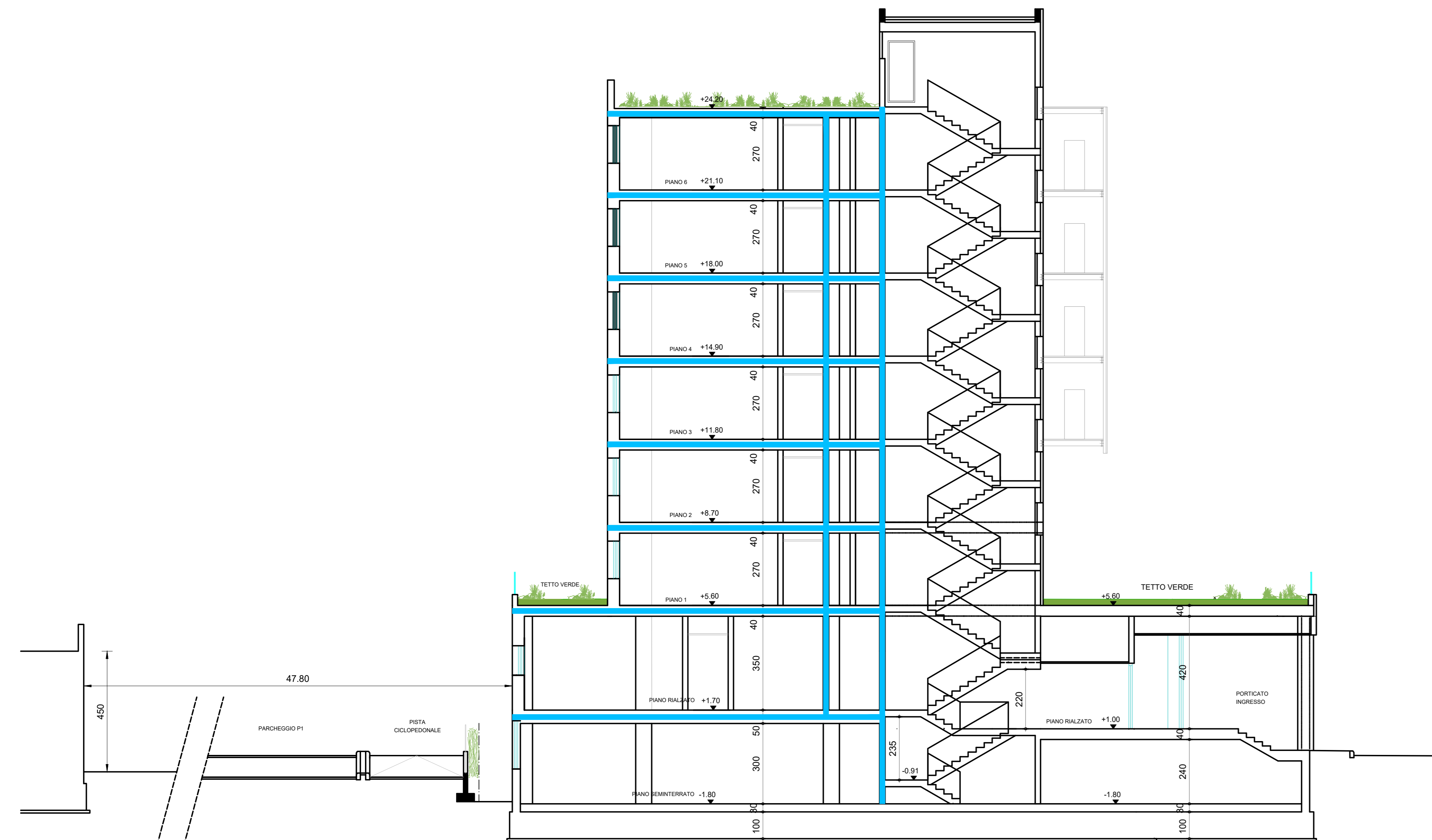
SEZIONE B-B
