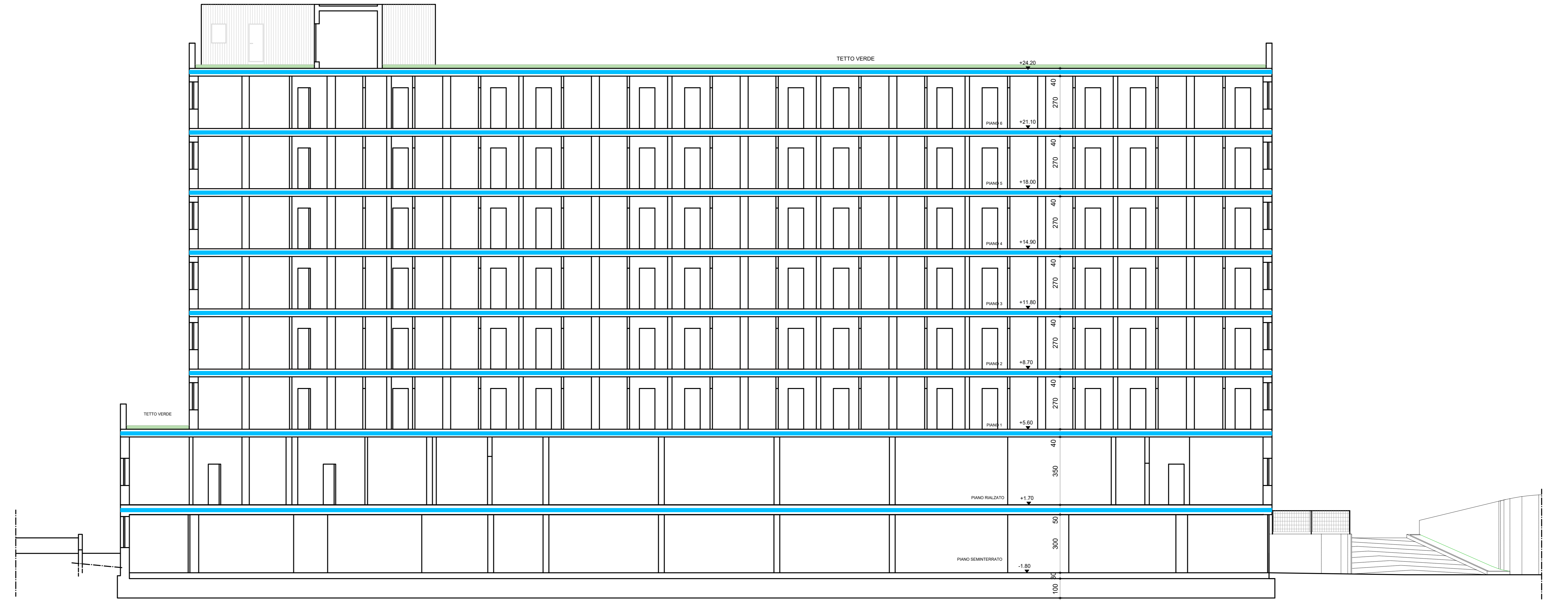
SEZIONE B-D
