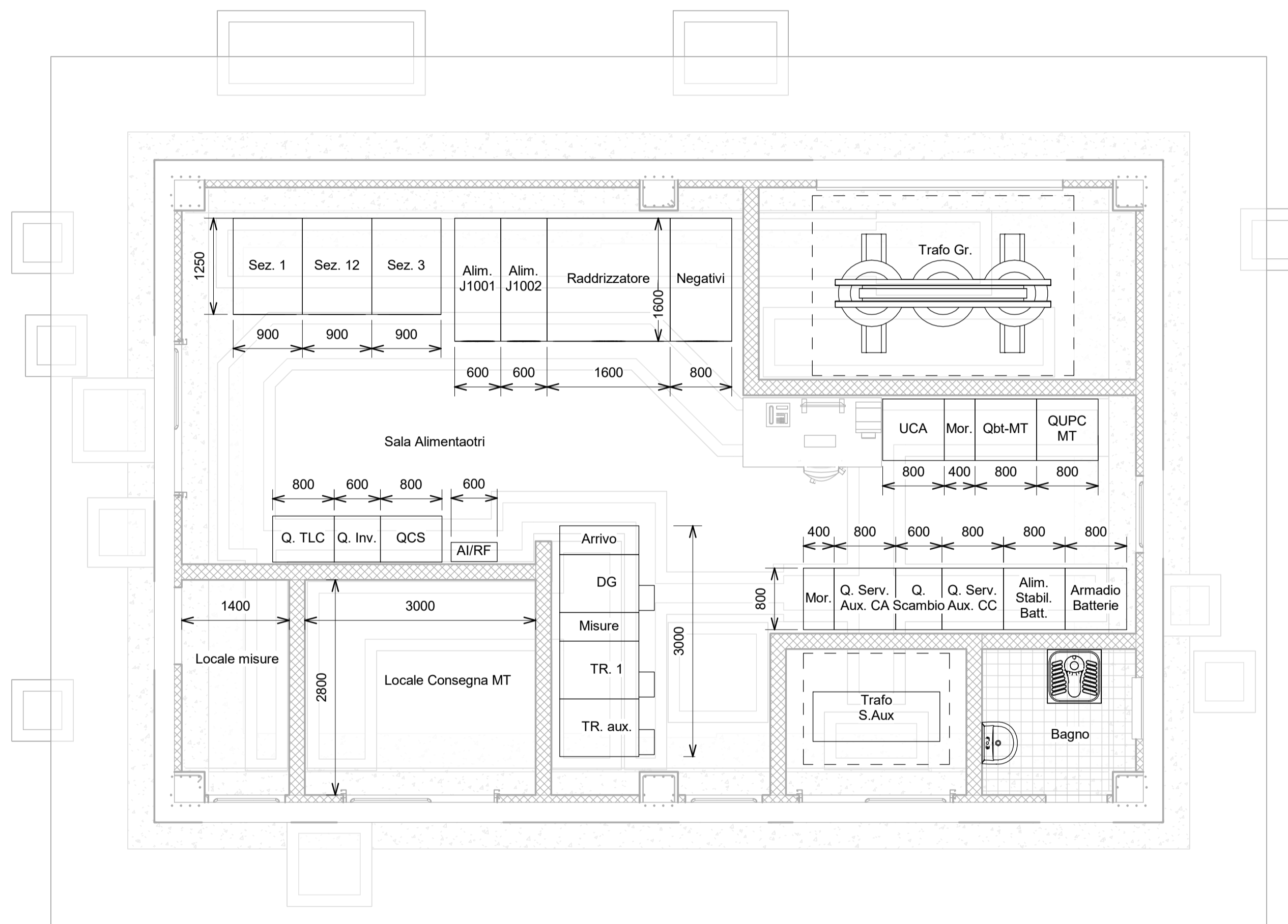
1 Disposizione apparecchiature (Layout) 1 : 50
