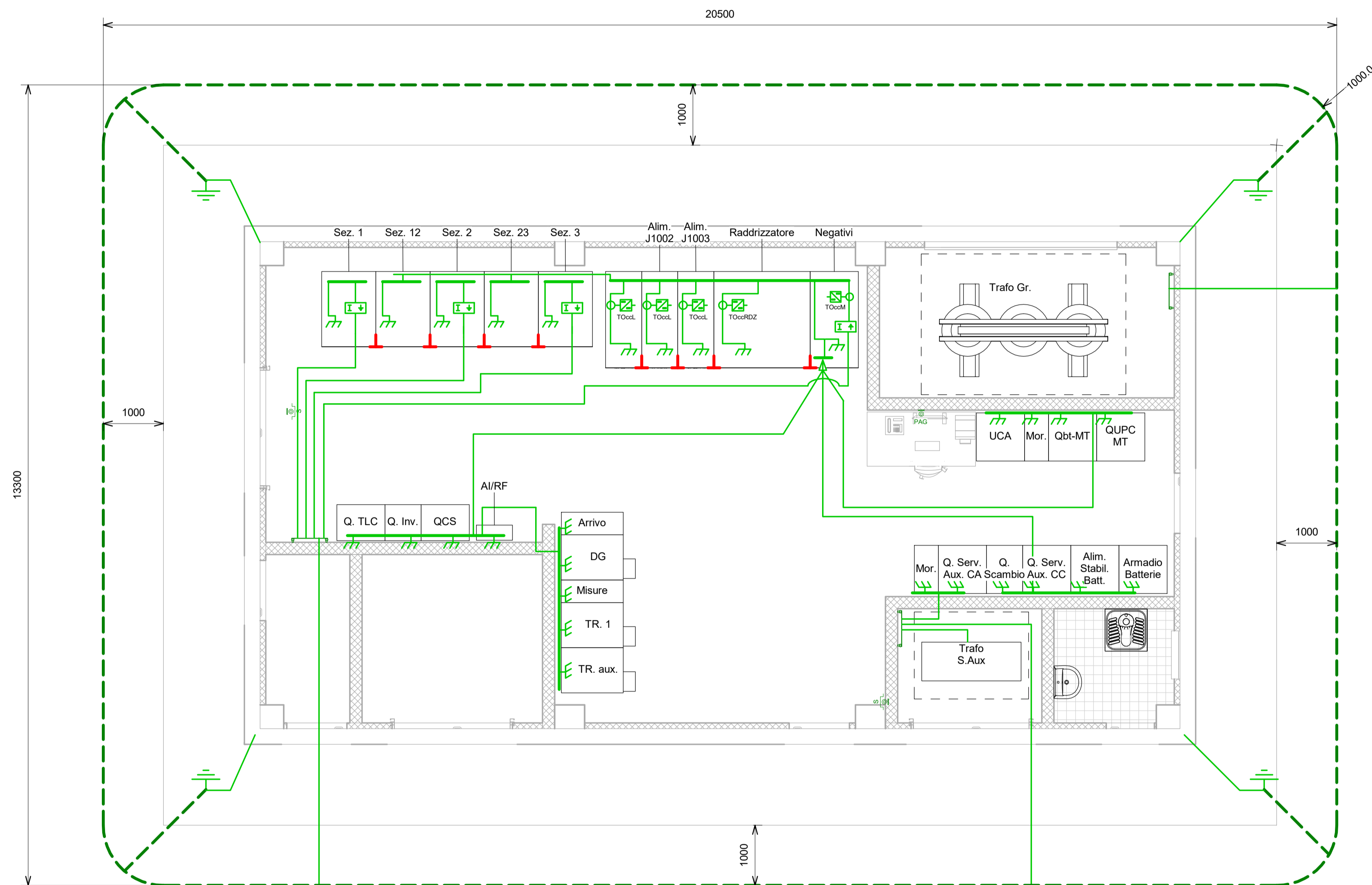
1 Impianto di Terra 1 : 50
