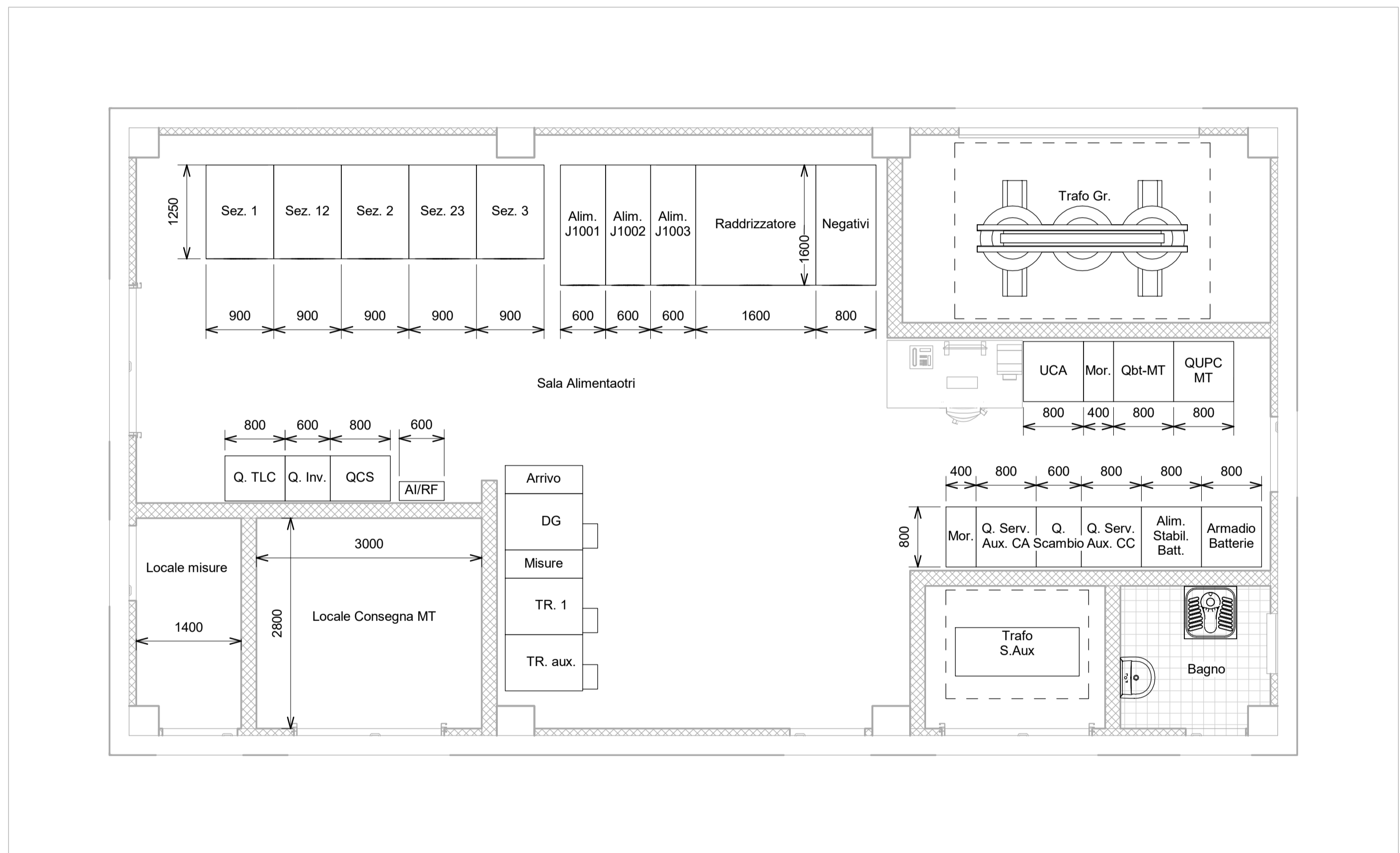
1 Disposizione apparecchiature (Layout) 1 : 50
