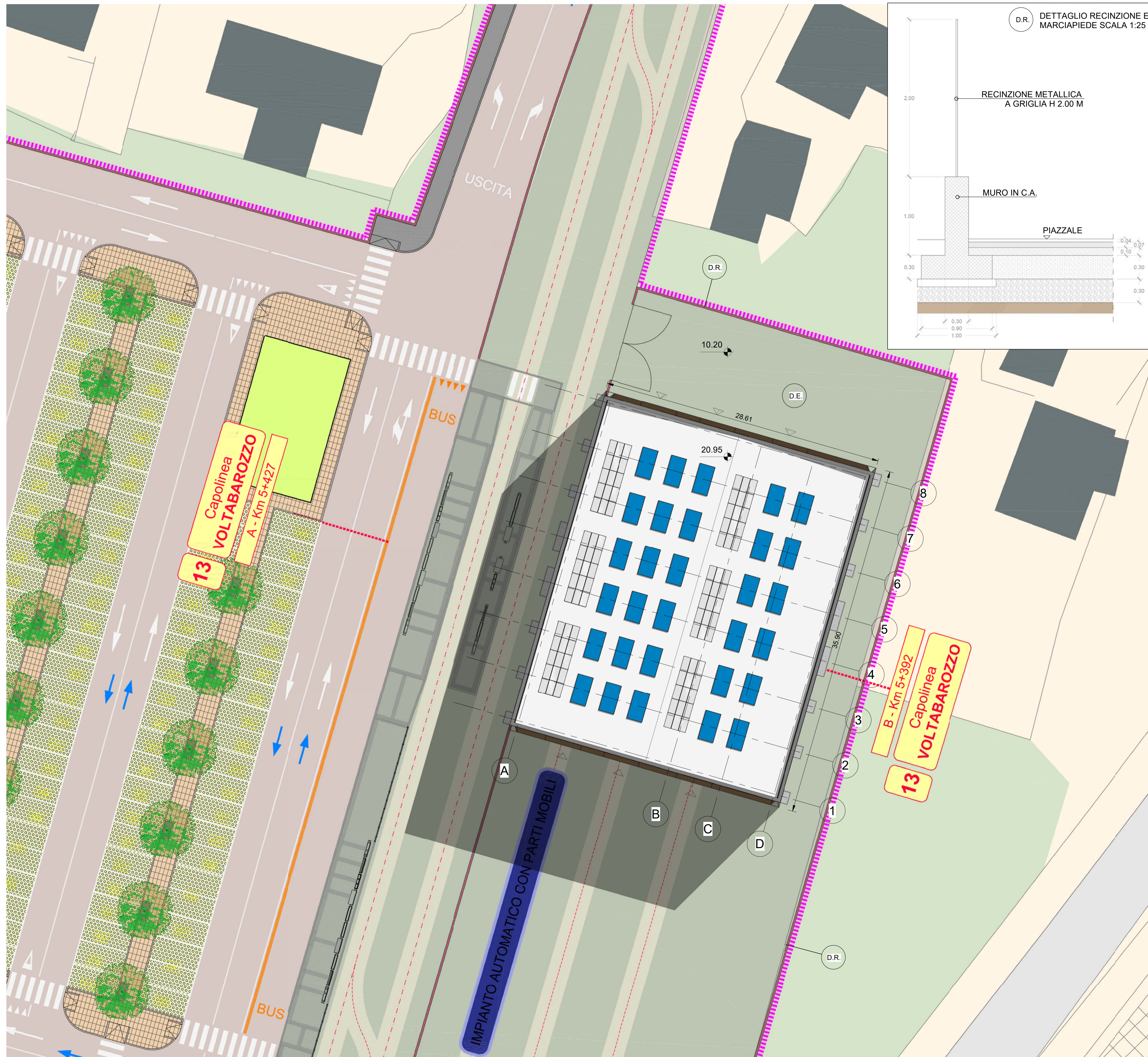
1 Planivolumetrico 1 : 200
