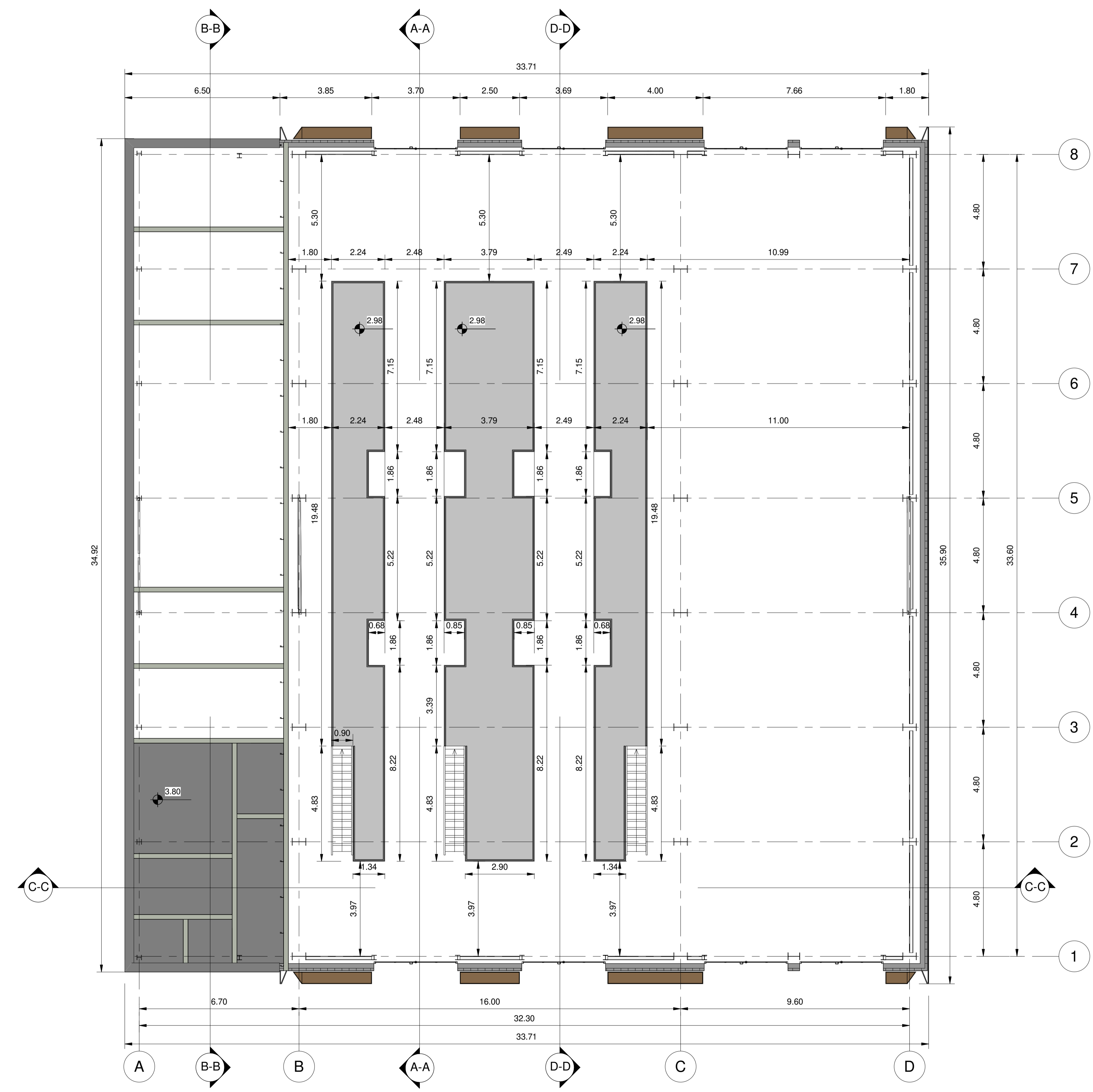
1 LPF - M1 Passerelle 1 : 100
