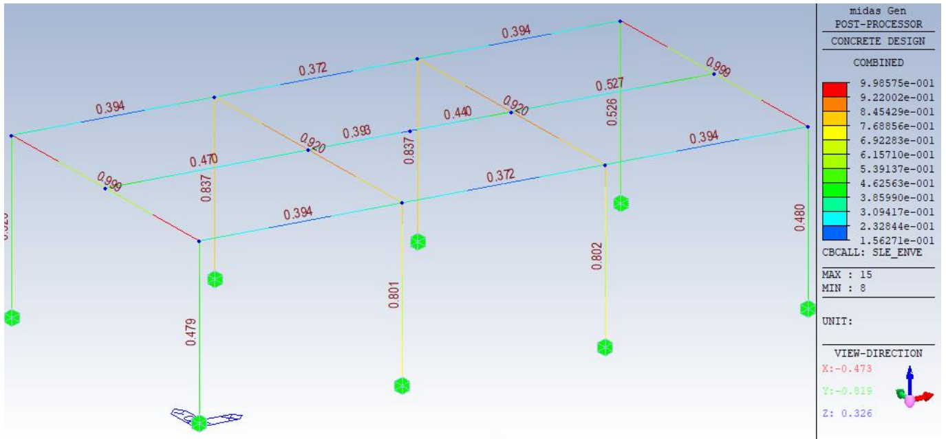
23. Verifica delle sezioni con relativi tassi di lavoro
