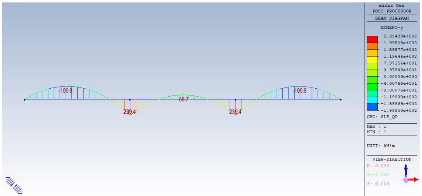
28. cLCB65 - Combinazione SLE Quasi permanente – Momento flettente M_y
