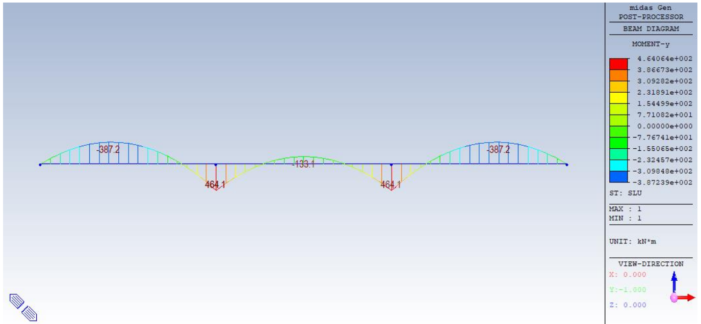
24. cLCB15 - Combinazione SLU – Momento flettente My
