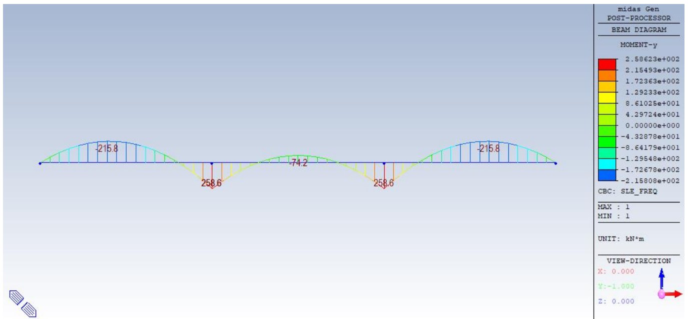
27. cLCB62 - Combinazione SLE Frequente – Momento flettente My
