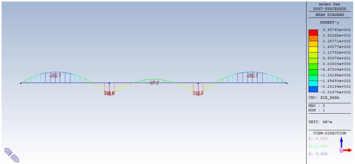
26. cLCB48 - Combinazione SLE Rara – Momento flettente My
