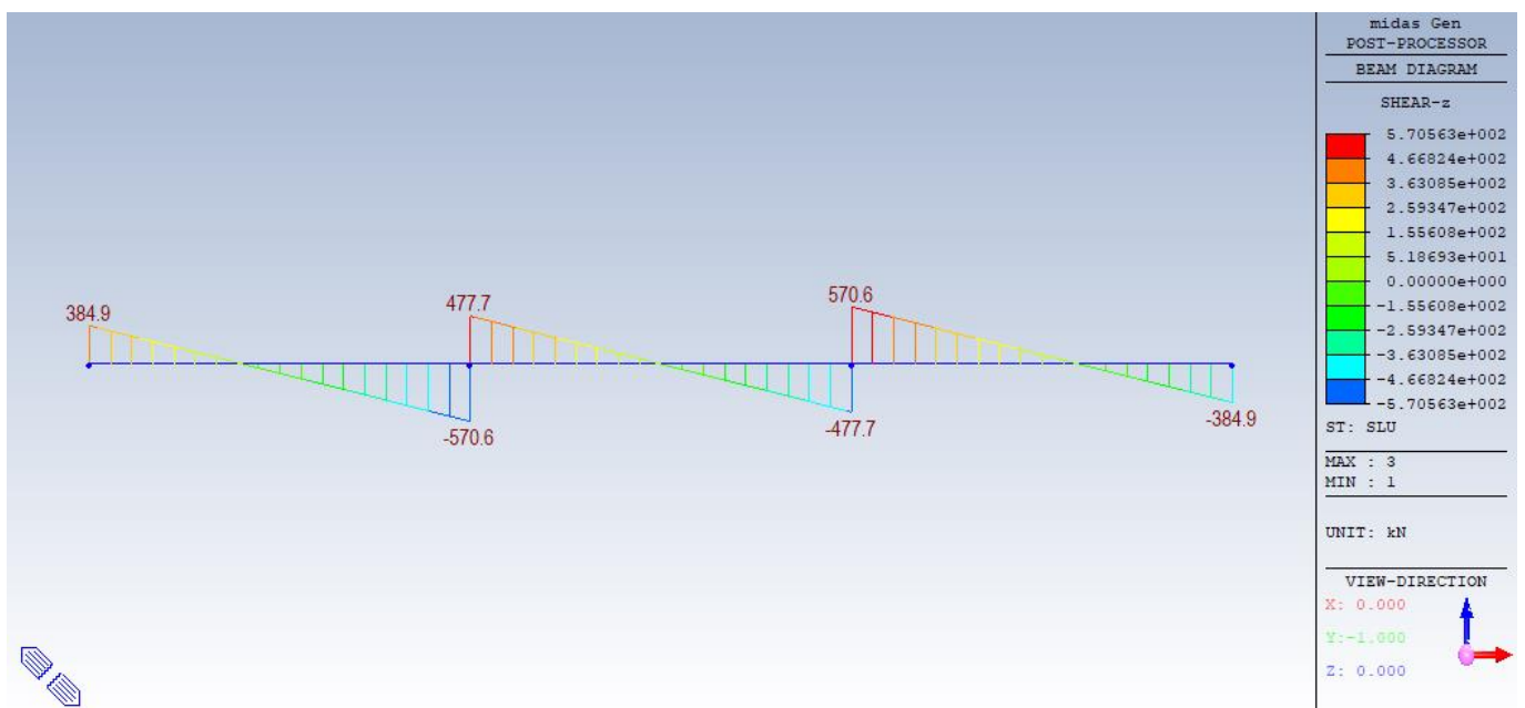
25. cLCB15 - Combinazione SLU – Taglio Fz
