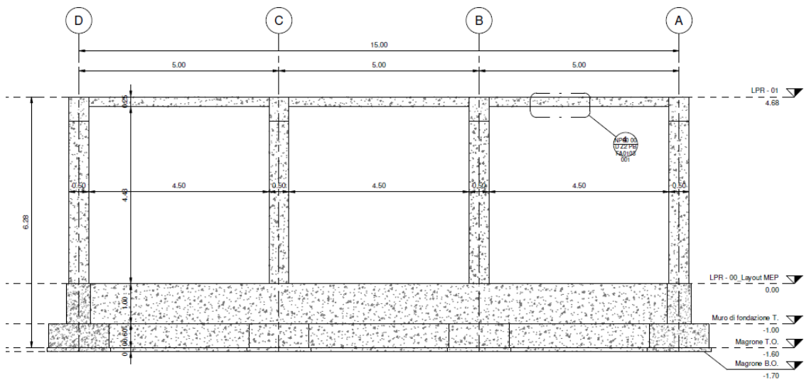
3. Sezione longitudinale
