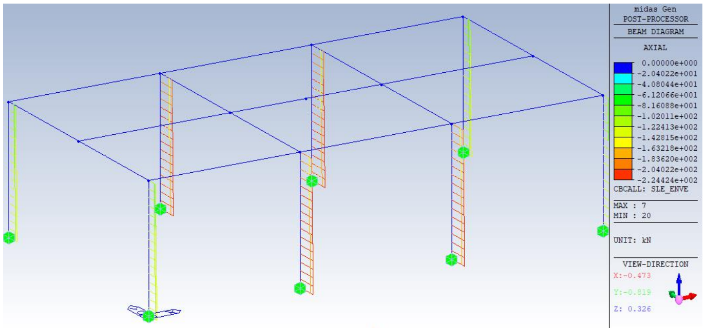
22. Enve SLE – Andamento degli sforzi assiali F_x
