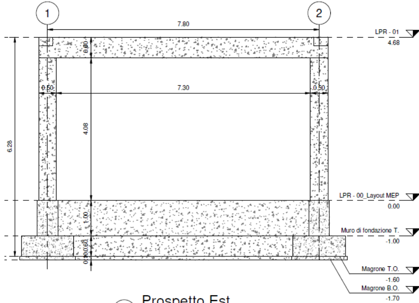
1 Prospetto Est 1 : 50
