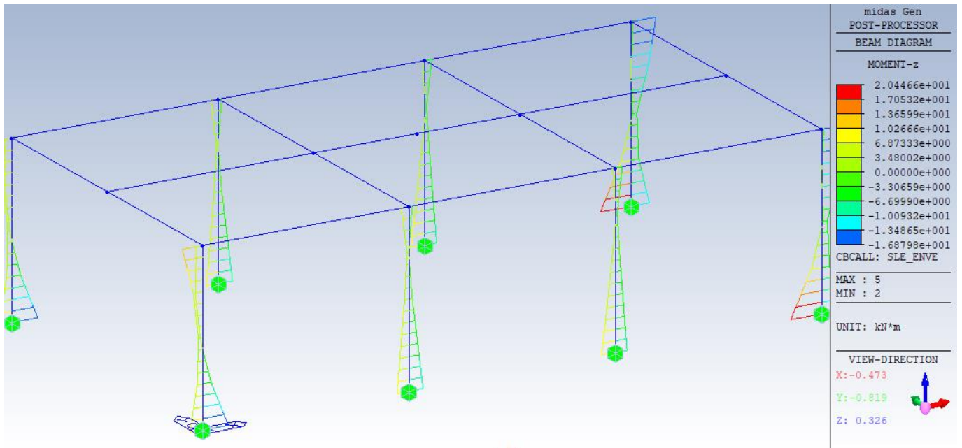
21. Enve SLE – Andamento dei momenti flettenti M_z
