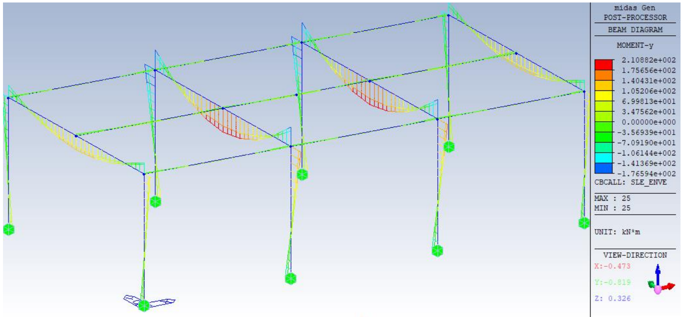
20. Enve SLE – Andamento dei momenti flettenti My
