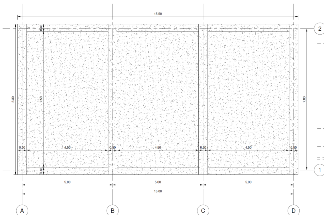
1. Pianta copertura
