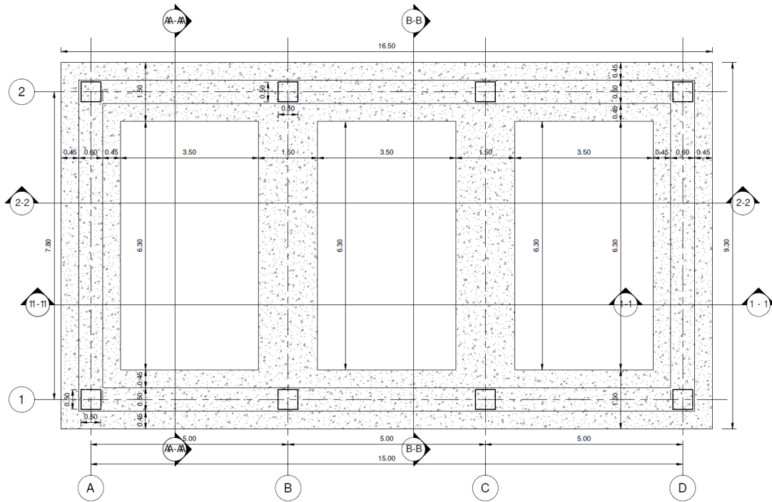
2. Pianta fondazioni
