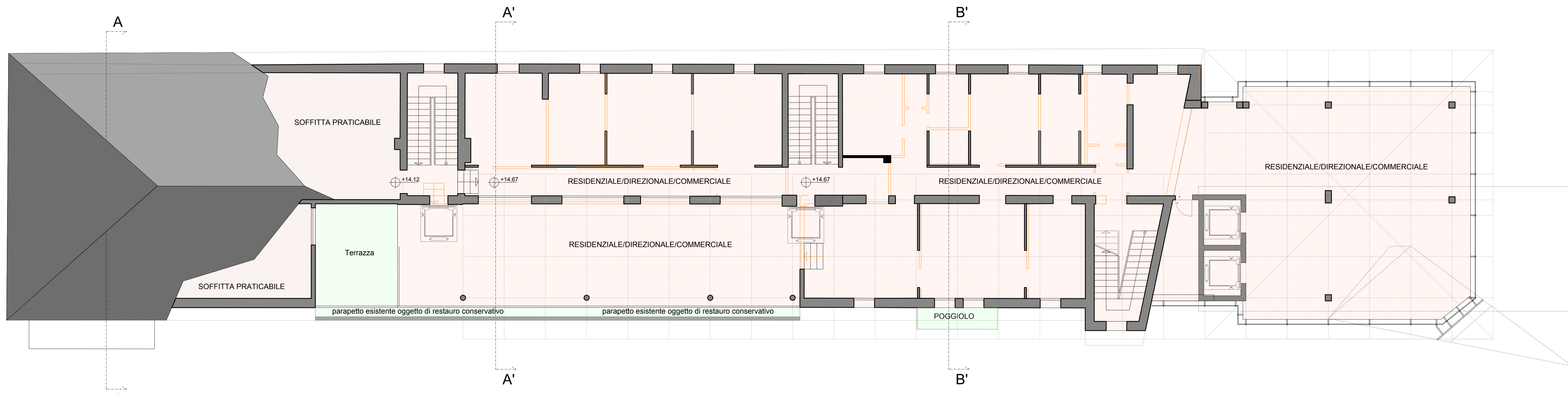
Pianta Piano Quarto Palazzina Ovest PROGETTO
