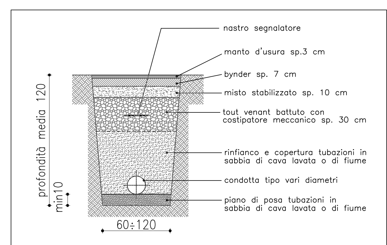
PARTICOLARE SCAVO TIPO PER CONDOTTE SCALA 1:20
