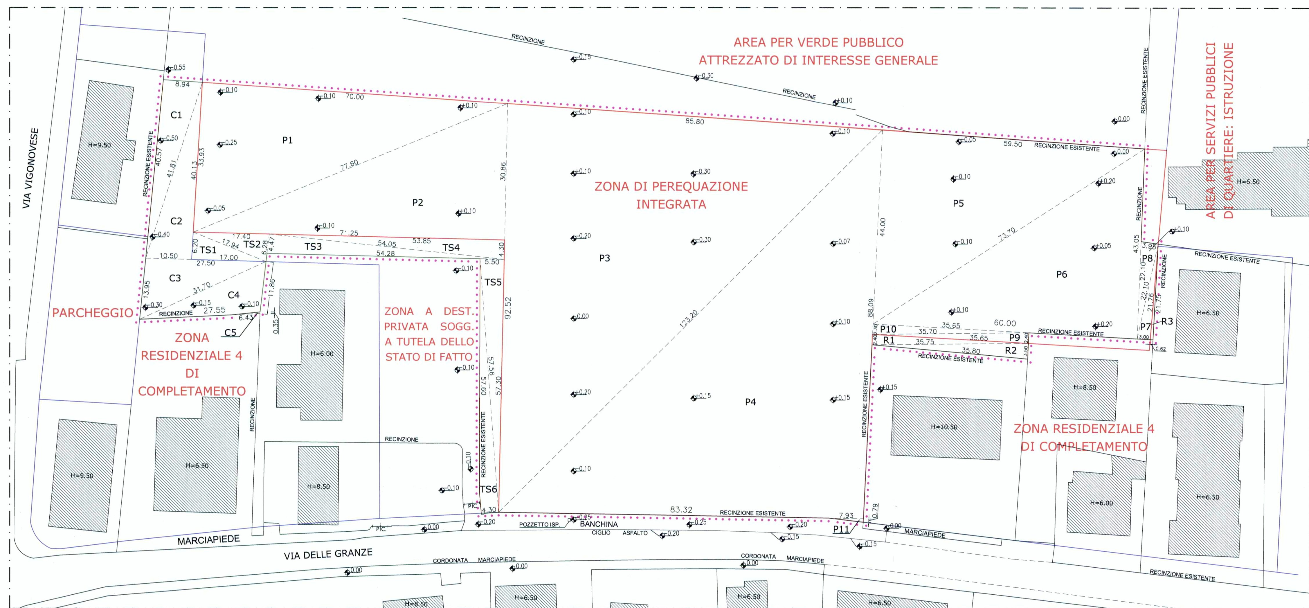
STATO DI FATTO: RILIEVO TOPOGRAFICO E PLANOALTIMETRICO
