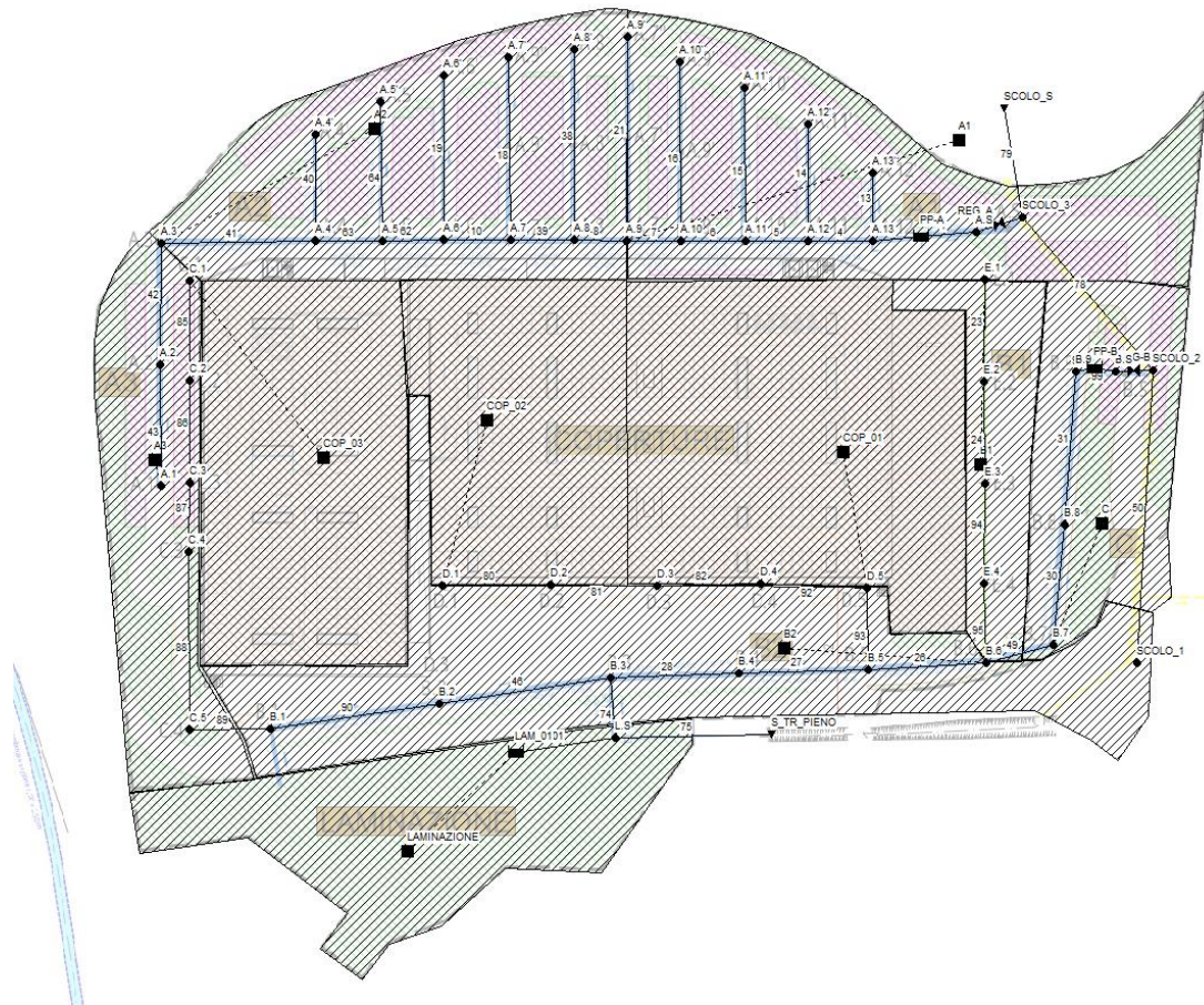
Figura 11: Rappresentazione del modello idrologico-idraulico
