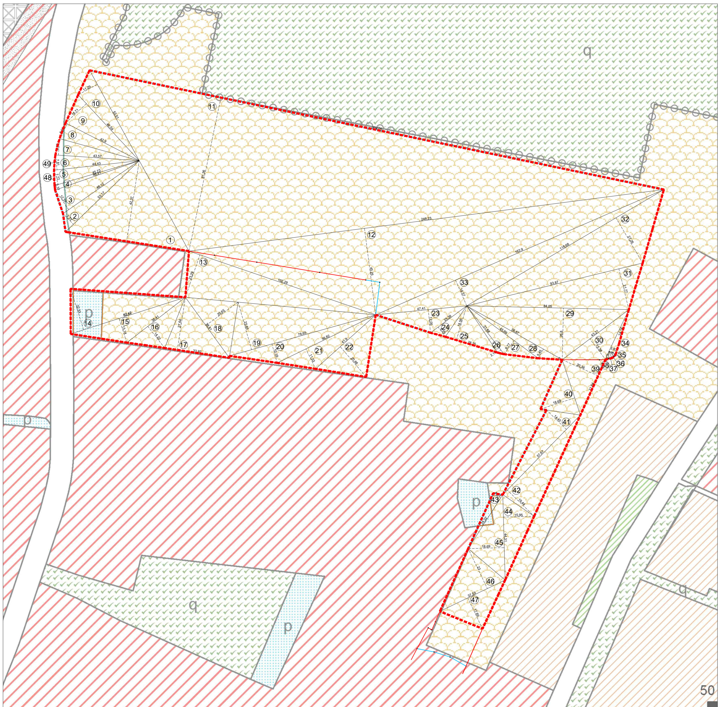
LETTURA DEL PIANO DEGLI INTERVENTI NELL'AMBITO DI INTERVENTO MODIFICATO - CALCOLO DELLE AREE DELL'AMBITO DI INTERVENTO MEDIANTE TRIANGOLAZIONE SCALA 1:1000
