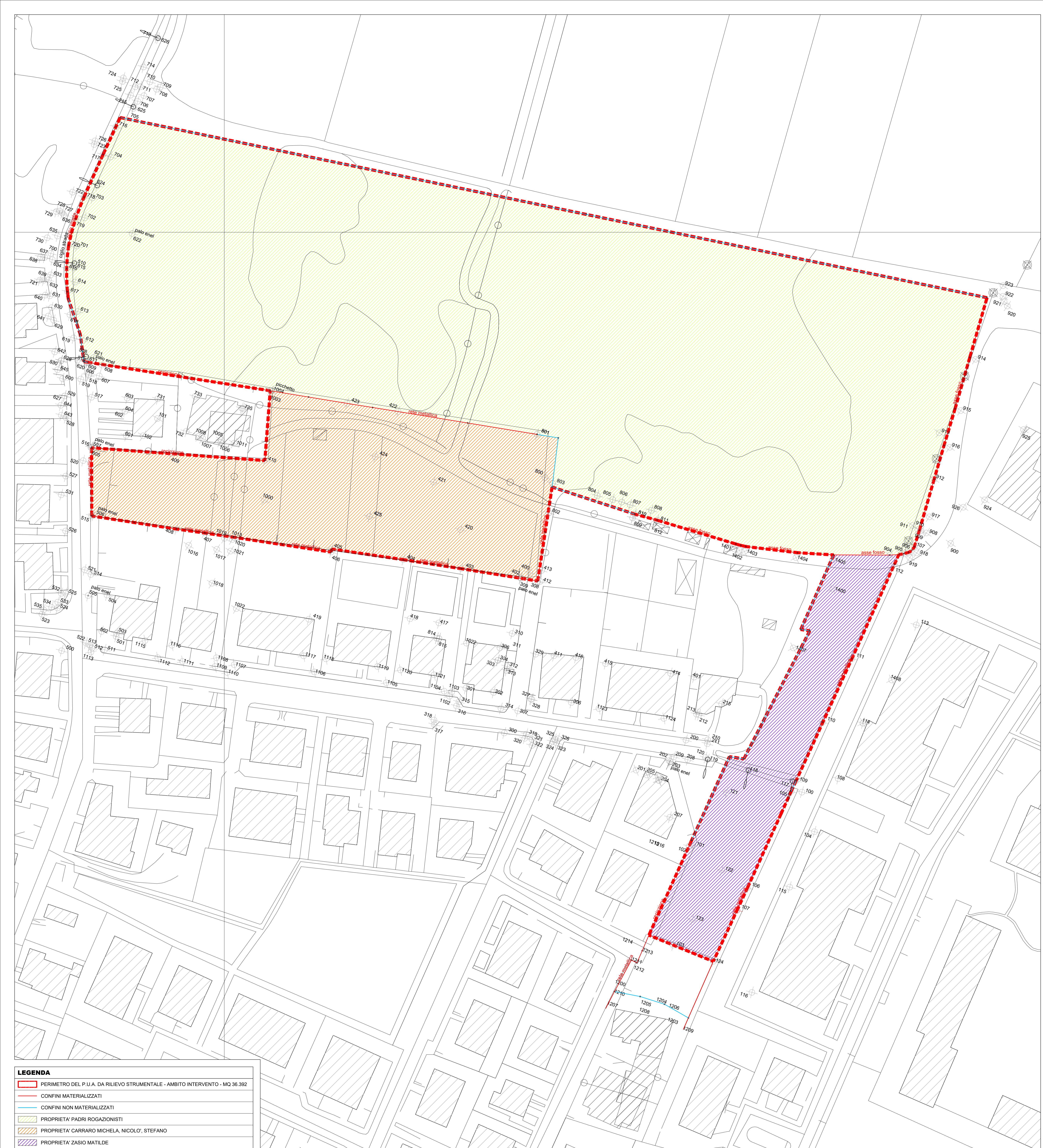
RILIEVO STRUMENTALE SCALA 1:500
