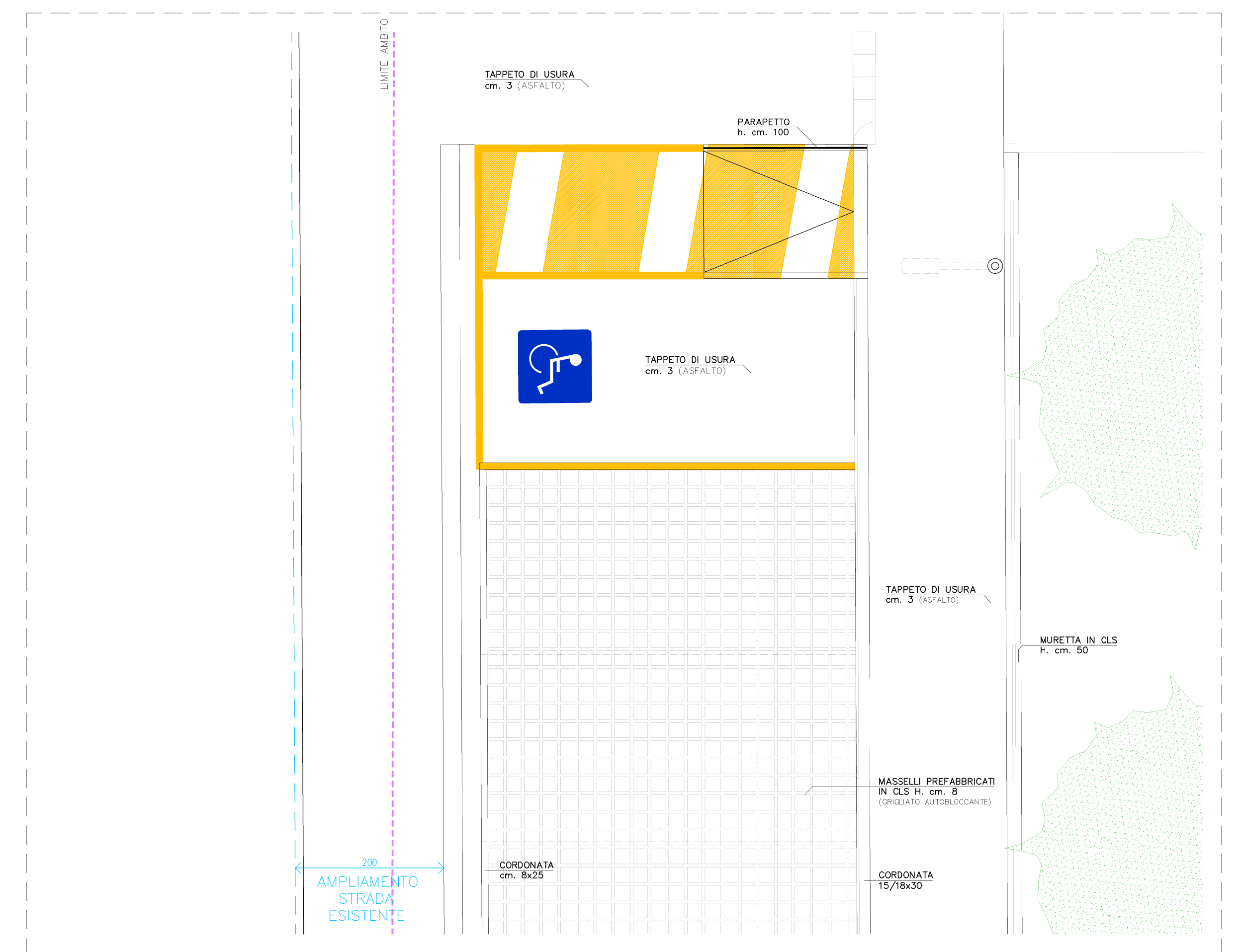
PARTICOLARE PIANTA MARGIAPIEDE - STRADA ③ SCALA 1:50
