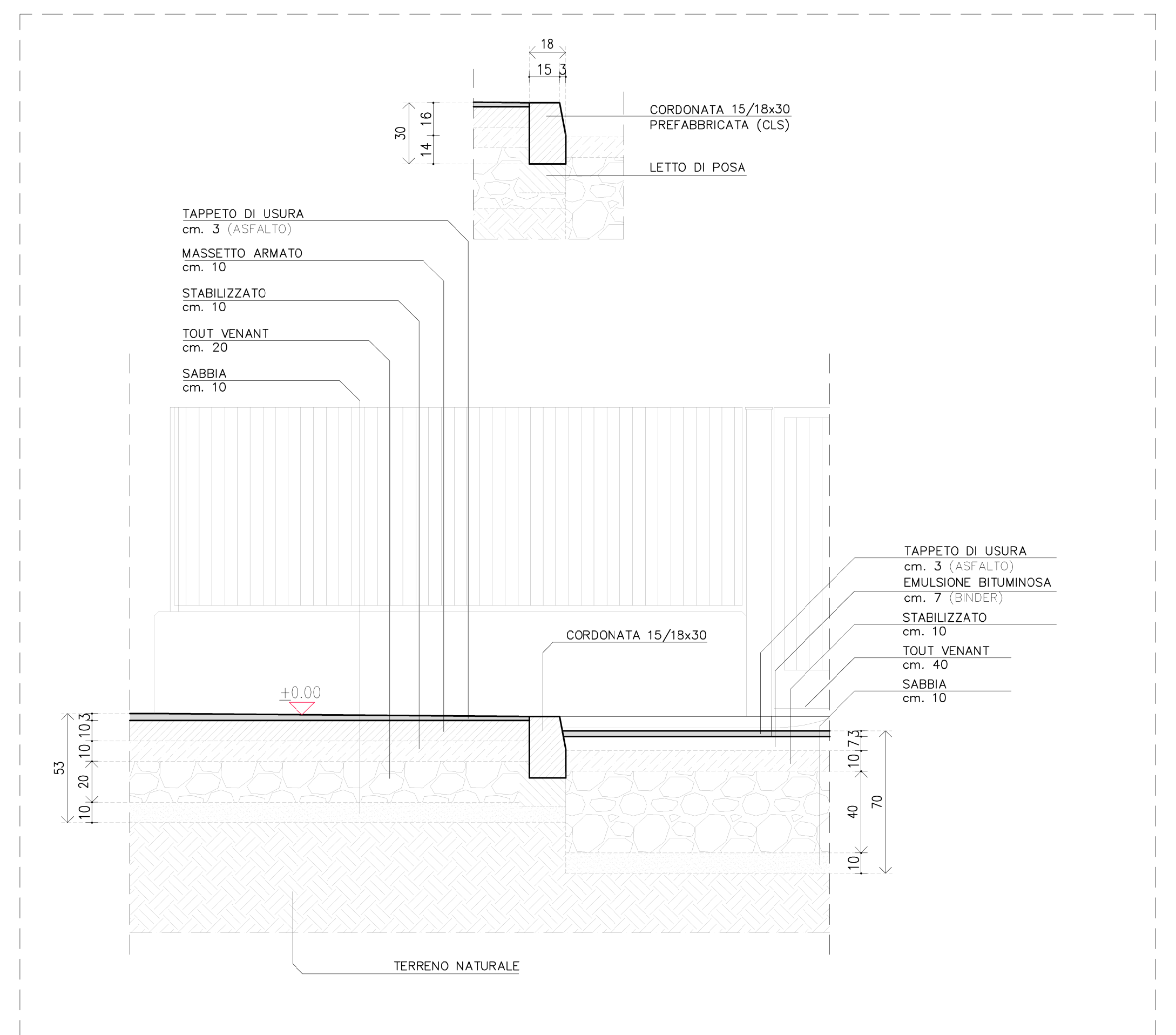
PARTICOLARE SEZIONE LONGITUDINALE MARGIAPIEDE - STRADA ③ SCALA 1:20
