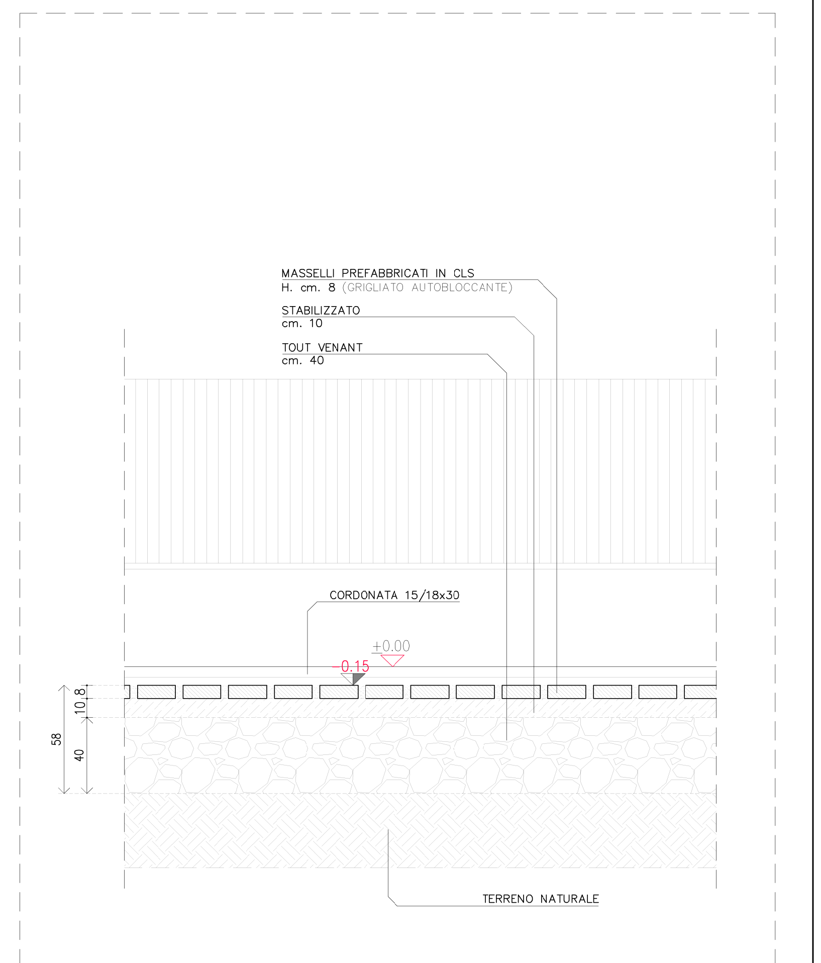
PARTICOLARE SEZIONE LONGITUDINALE PARCHEGGI ③ SCALA 1:20
