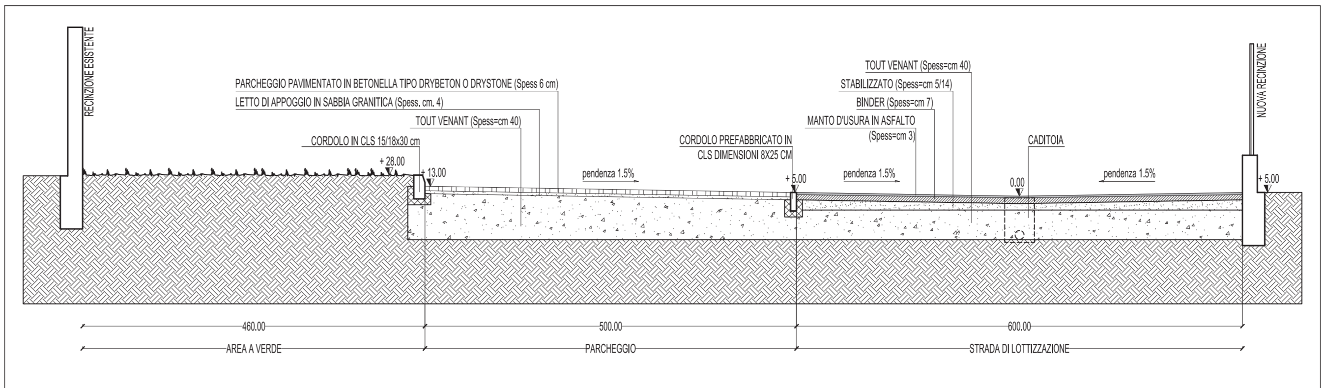
SEZIONE TRASVERSALE A - A' SCALA 1:50
